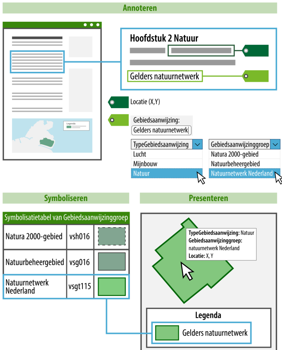
Figuur 3 Presentatiemodel: annoteren met object, type en groep, in combinatie met symbolcode uit waardelijst IMOW, toepassing standaardweergave
