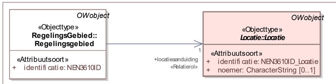
Figuur 46 Uitsnede uit IMOW-diagram voor objecttype Regelingsgebied
